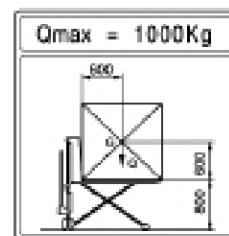
Рис. 10: Размещение груза
