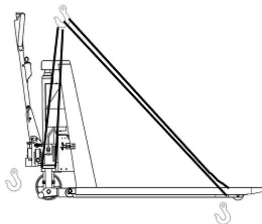
Рис. 9: Подъем тележки
