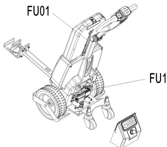
Рис. 18: Расположение предохранителей
