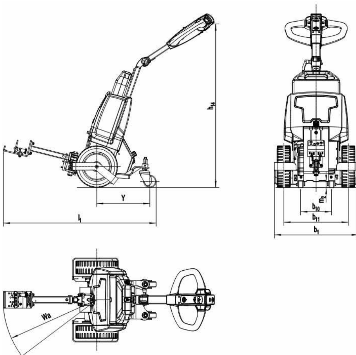
Рис. 2: Схематический чертеж конструкции
