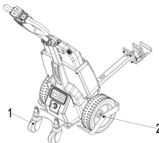
Рис. 17: Точки смазки
