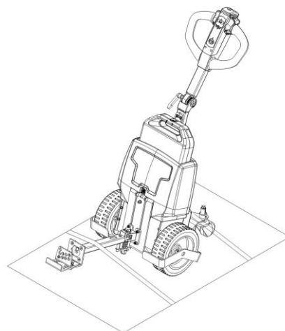
Рис. 6: Точки крепления
