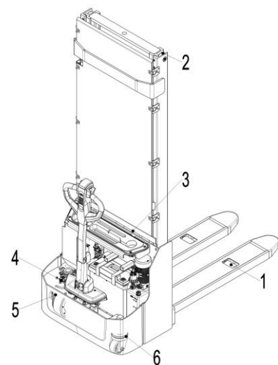
Рис. 16: Точки смазки
