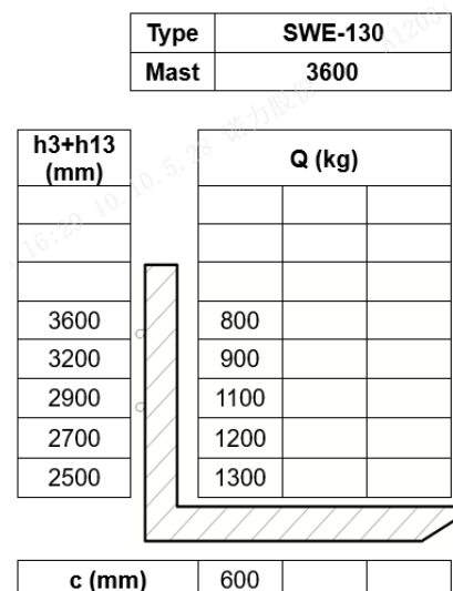
Рис. 9: Остаточная грузоподъемность
