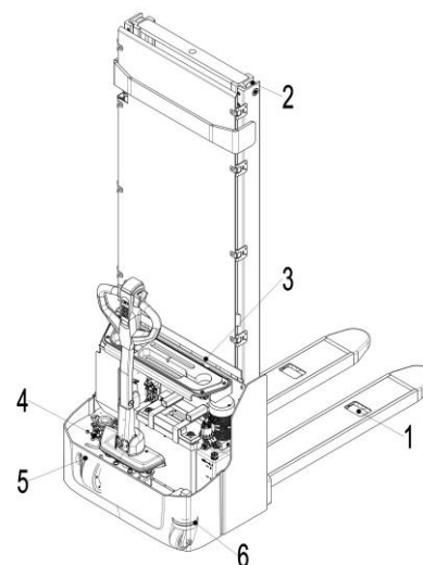
Рис. 16: Точки смазки
