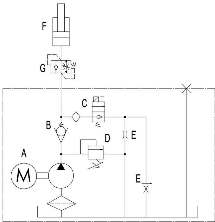
Рис. 19: Гидравлическая схема
