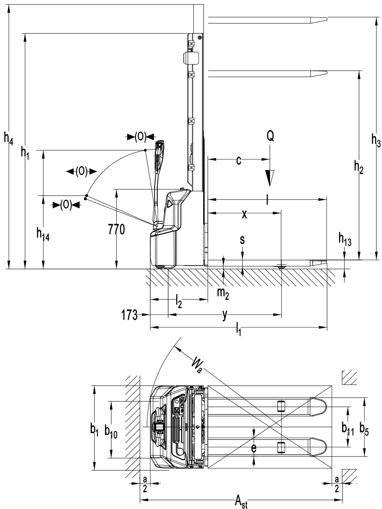
Рис. 2: Технические характеристики
