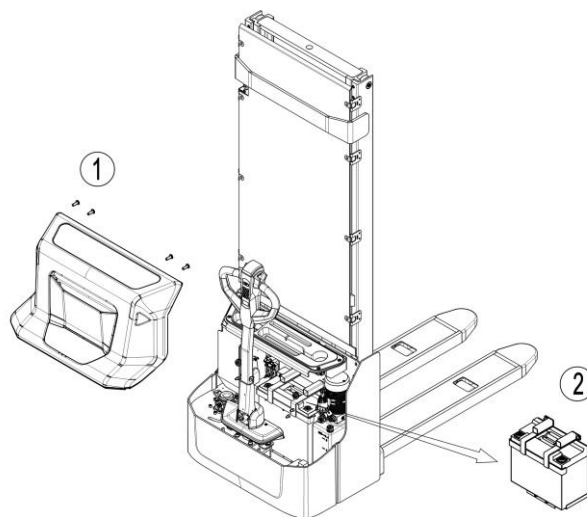
Рис. 15: Замена АКБ
