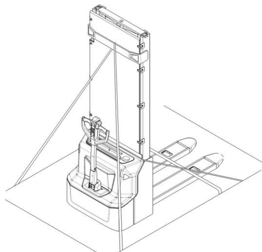
Рис.6: Точки фиксации
