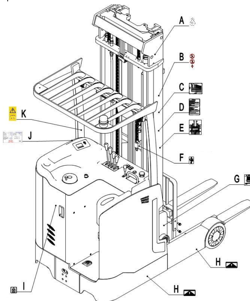
Рис. 3: Предупреждающие таблички
