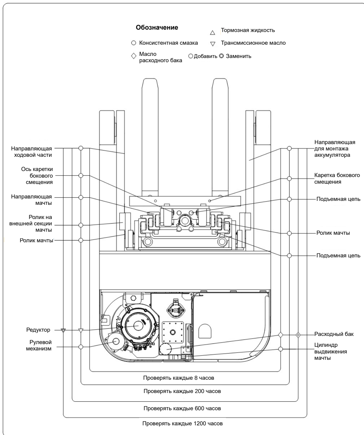
Рис. 17: Места для смазки
