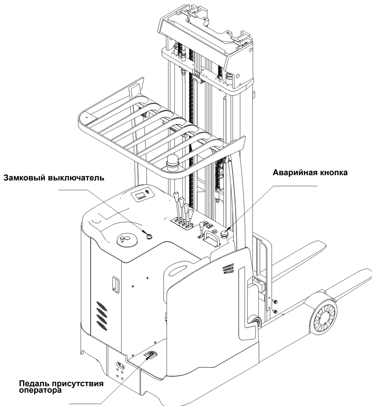
Рис. 4: Предохранительные устройства
