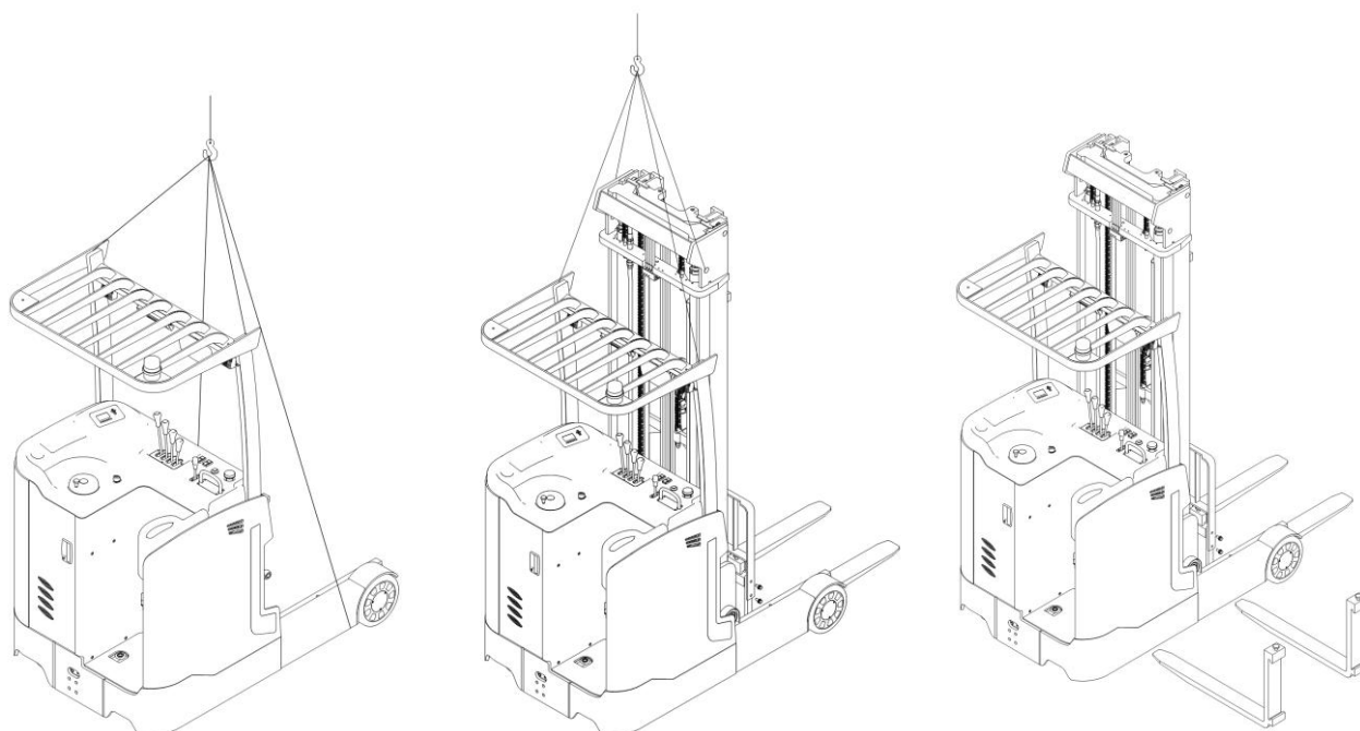
Подъем ходовой части ричтрака
