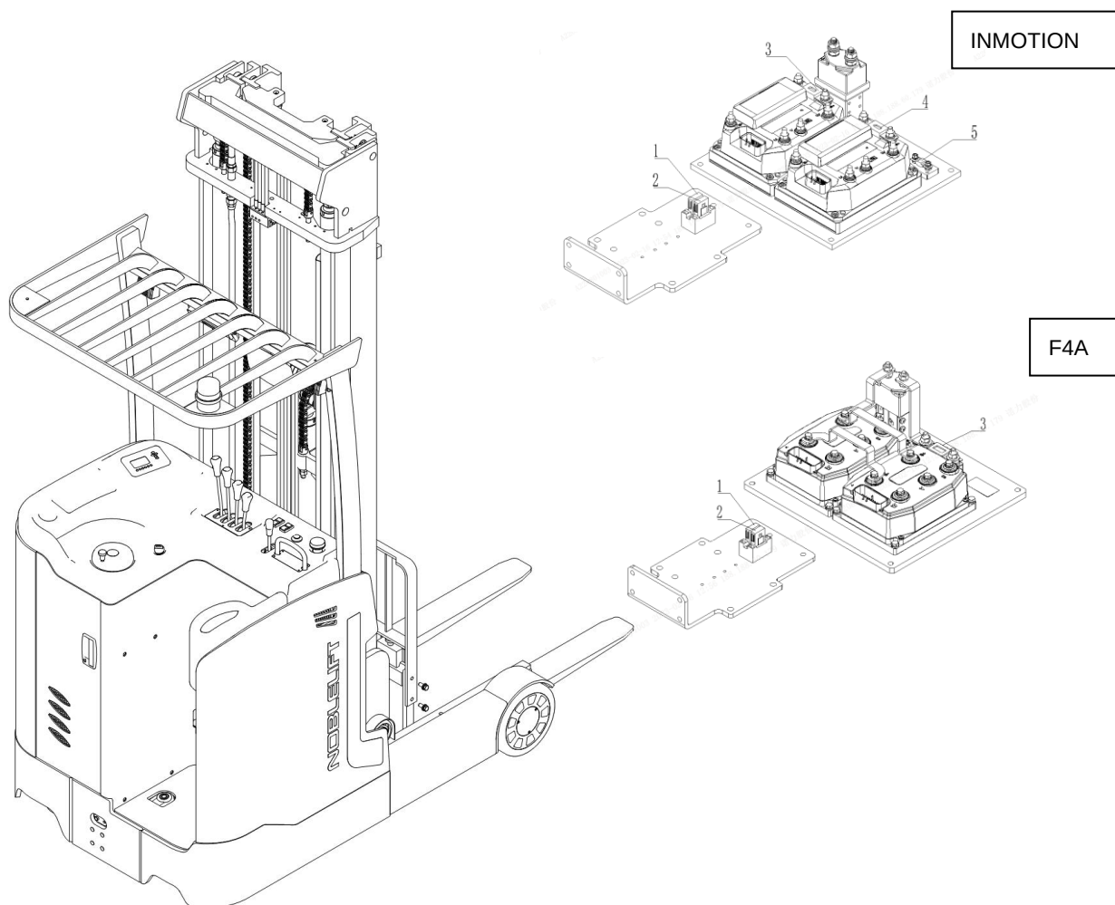
Рис. 18: Расположение предохранителей
