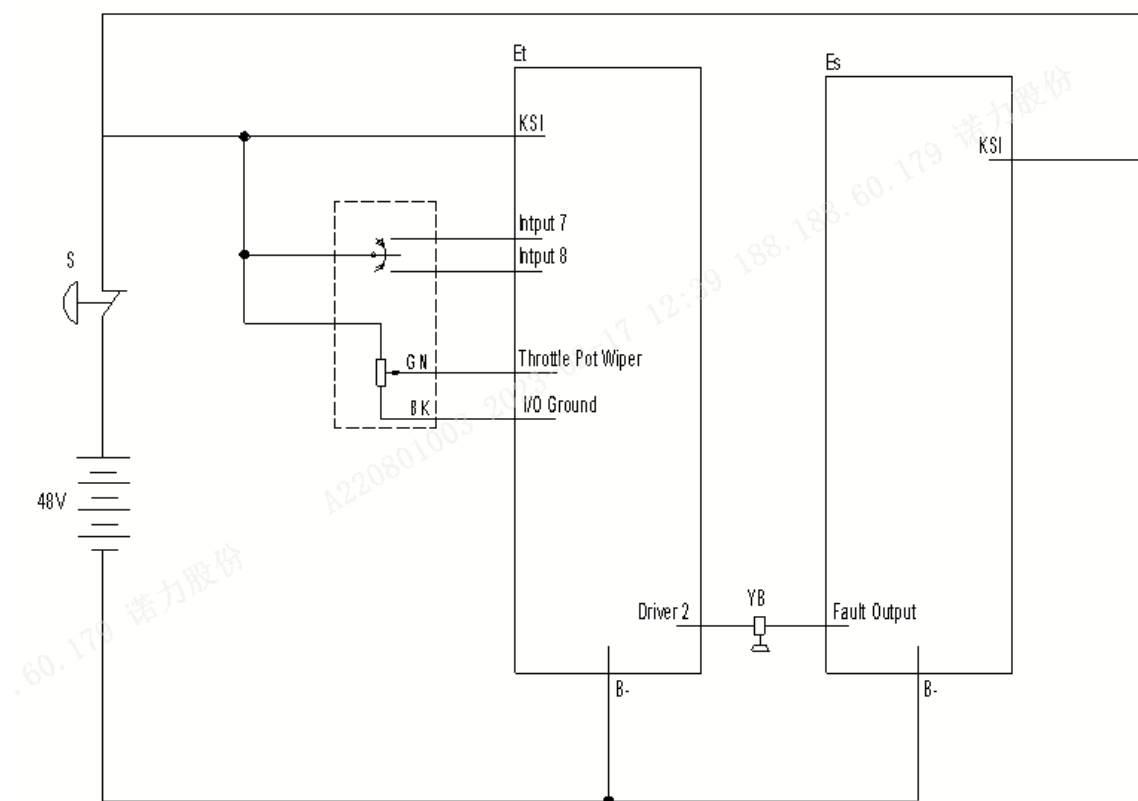
Рис. 20: Схема тормозной системы – CURTIS (парковочный тормоз)
