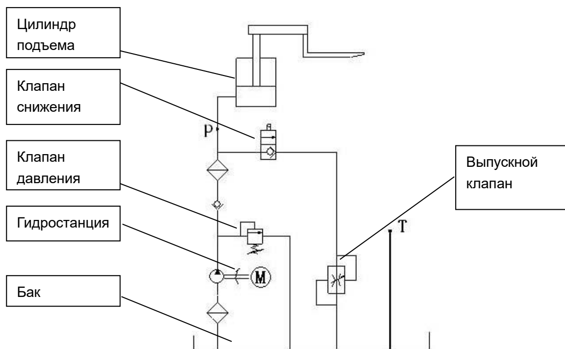
Рис. 17: Гидравлическая система
